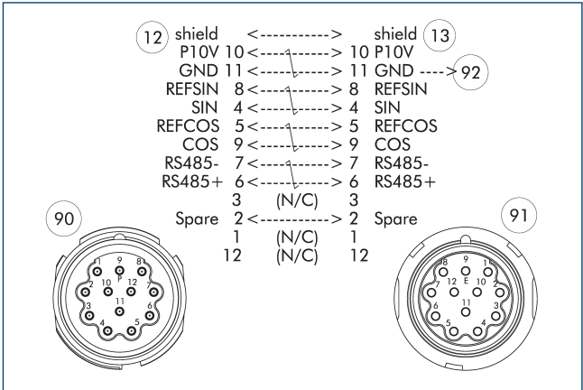
12 Côté maître 91 Interface JAE 13 Côté adaptateur 92 contact avancé 90 Interface JAE
